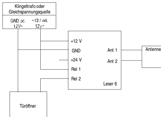
Schaltungsbeispiel Türöffner:
